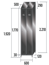
SV-30/2 INOX COD: 83902 49kg · 0,69m 3
